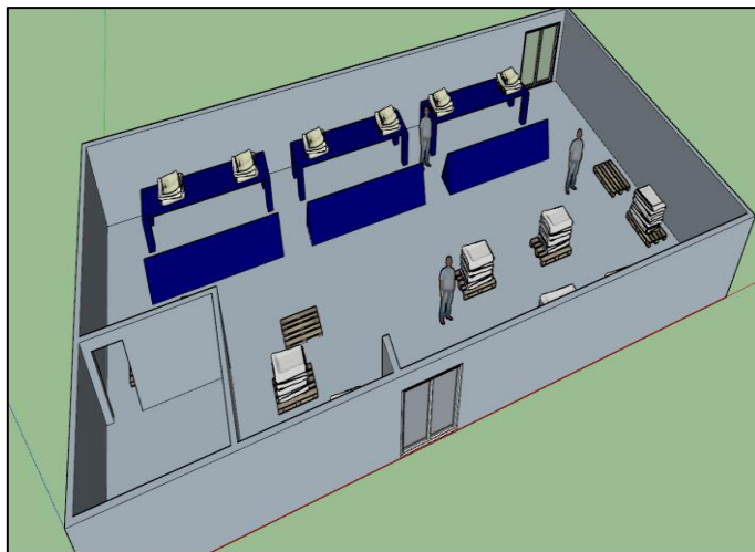
Figura 2: Layout Atual do Setor de Classificação no formato 3D. Fonte: Autores, (2018).
