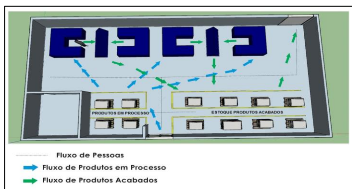
Figura 3: Planta baixa do novo layout.
