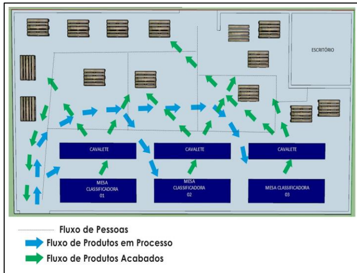
Figura 1: Layout Atual do Setor de Classificação. Fonte: Autores, (2018).
